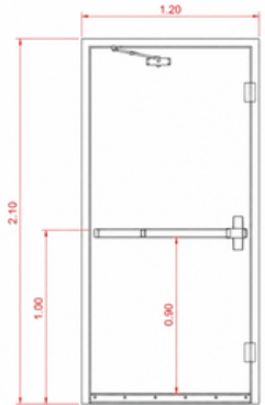
Plano y dimensiones
